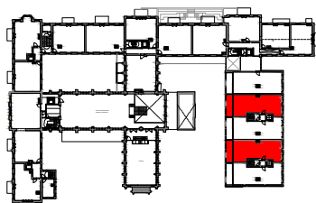
grondplan verdieping 1 - nieuwe toestand
