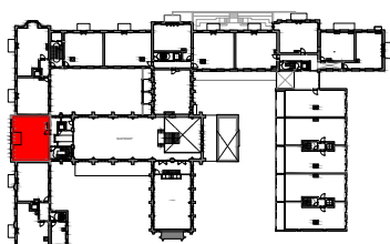
grondplan verdieping 1 - nieuwe toestand
