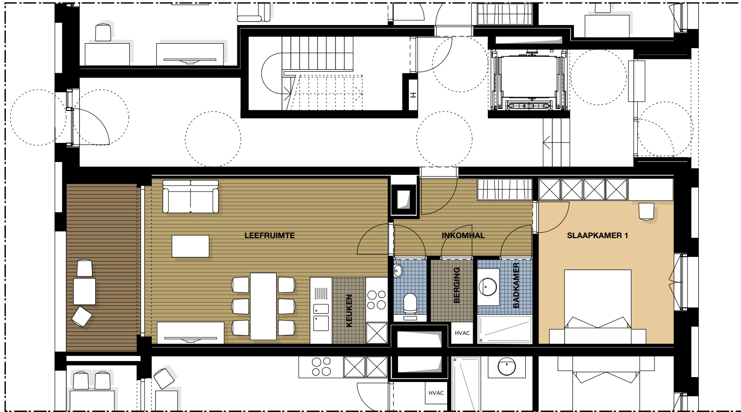
appartement 0AL
